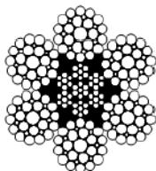
【正】表 2.2.4 ワイヤロープ IWRC 6×Fi (29) の破断力の例 (JIS G 3525-2013 による)
