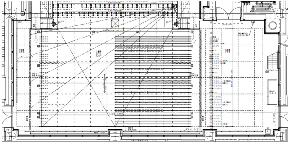
中劇場舞台機構 平面図
