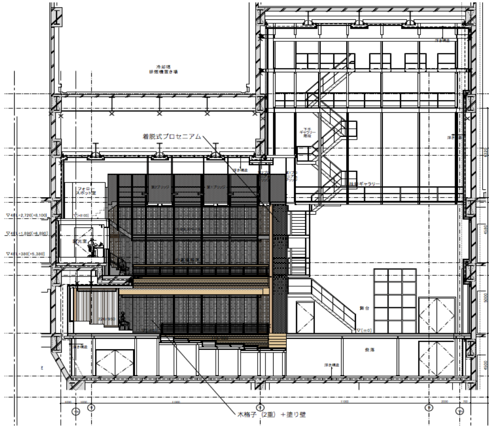
長手展開図
